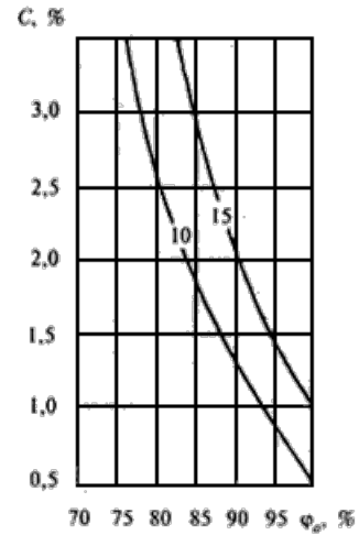
Рисунок Щ.5 - Изолинии сорбционного влагосодержания керамзитобетона \rho_0 = 1200 \text{ кг/м}^3 , содержащего \text{NaCl} - 50\% , \text{KCl} - 30\% , \text{MgCl}_2 - 10\% , при изменении относительной влажности воздуха \varphi_a, \% , и массового соледоержания C, \% , в стенах цехов дробления руды
