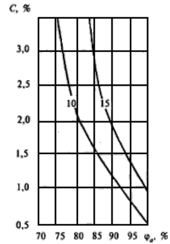
Рисунок Щ.4 - Изолинии сорбционного влагосодержания керамзитобетона \rho_0 = 1200 \text{ кг/м}^3 , содержащего \text{NaCl} - 60%, \text{KCl} - 30%, \text{MgCl}_2 - 10%, при изменении относительной влажности воздуха \varphi_a , %, и массового солесодержания C , %, в стенах флото-фабрик
